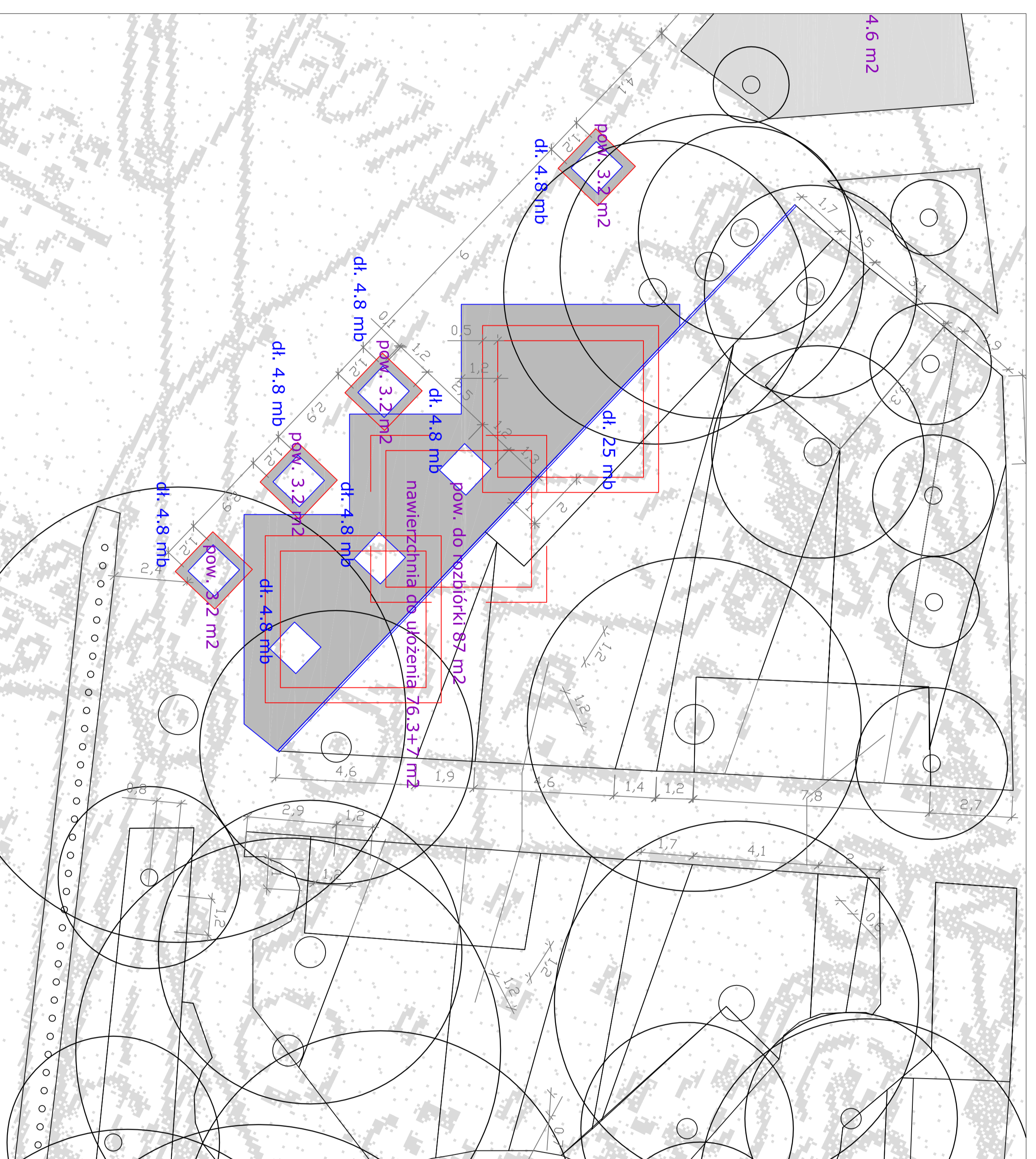
Rozbiórka istniejącej nawierzchni pod wiadami do zakresu ułożenia nowej nawierzchni
