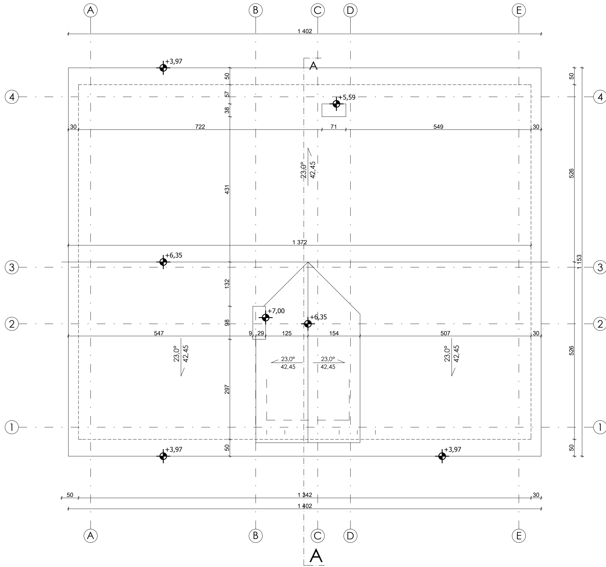
RZUT DACHU
