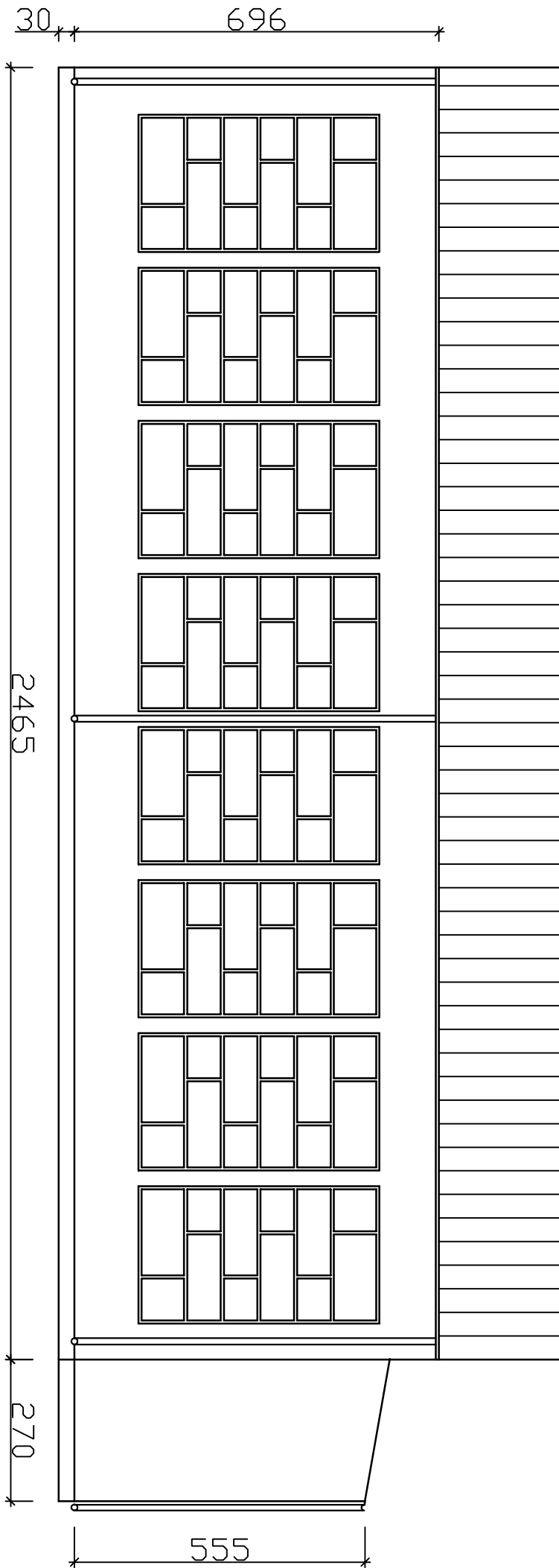
ELEWACJA TYLNA SALA GIMNASTYCZNA
