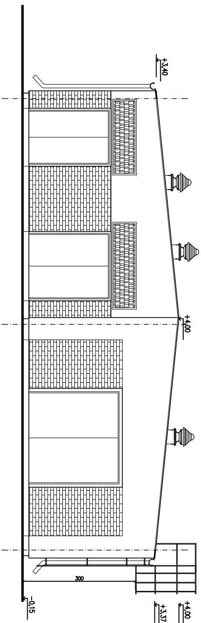
ELEWACJA WSCHODNIA
